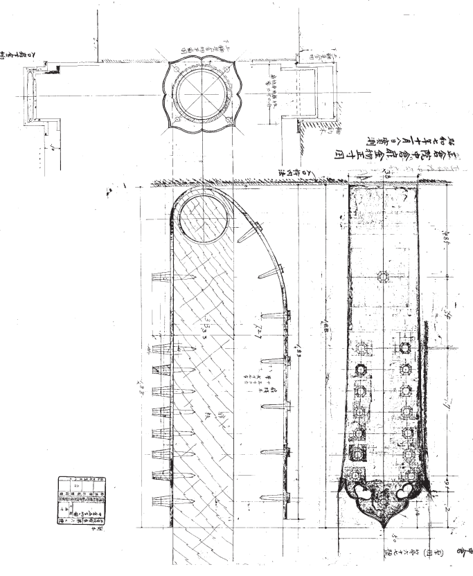
139 第六六号 正倉院宝庫南倉扉金物之図
