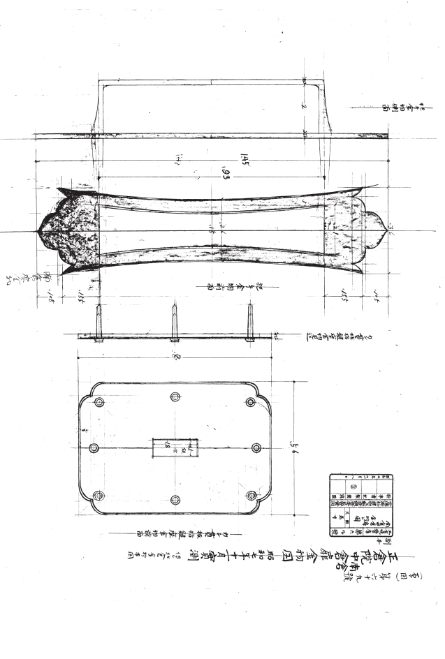
142 第六九号 正倉院宝庫南倉中倉扉金物之図
