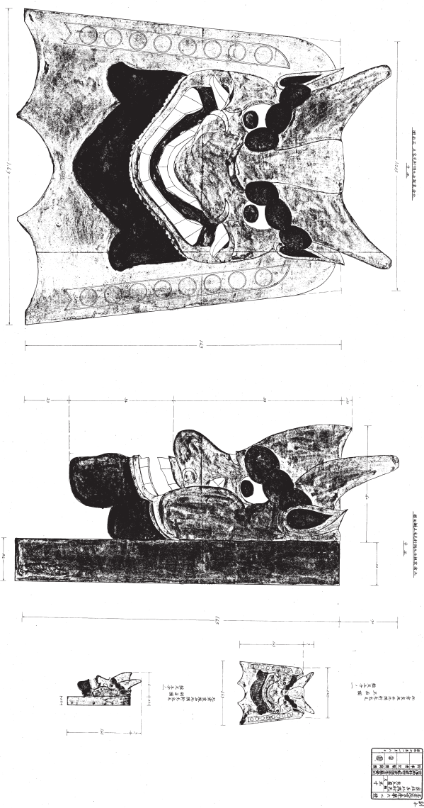
135 第六二号 正倉院宝庫西北隅軒先鬼瓦之図
