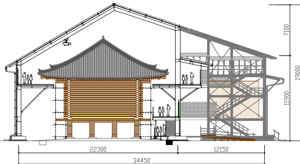
素屋根断面図
