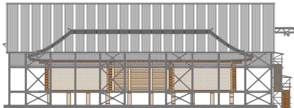
素屋根西立面図
