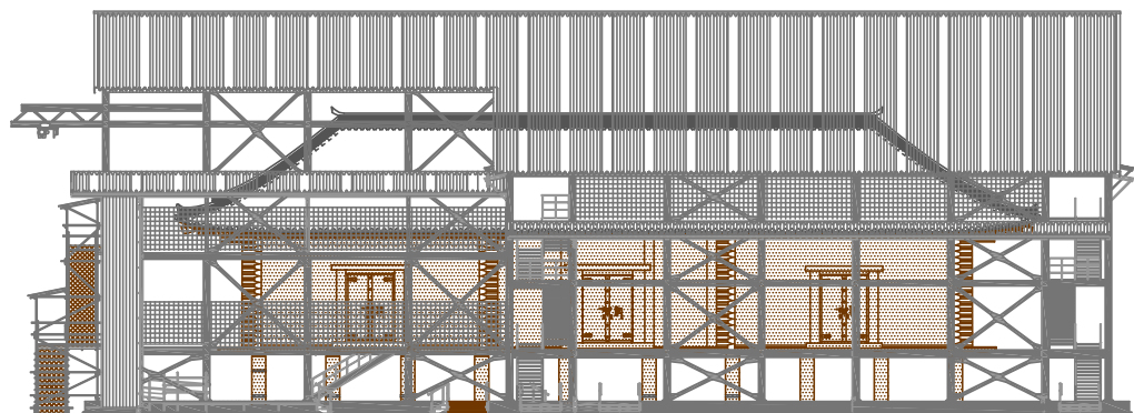
素屋根東立面図
