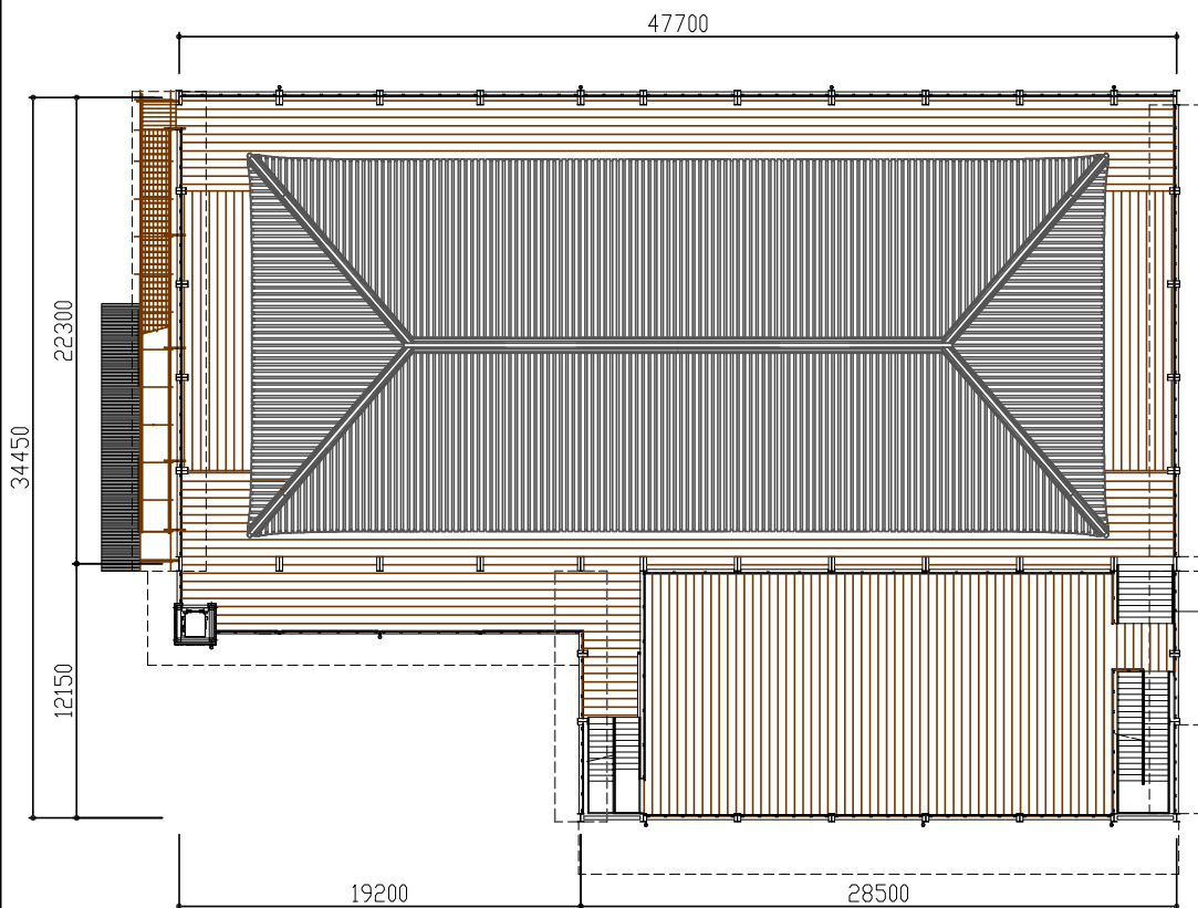
素屋根 3階平面図
